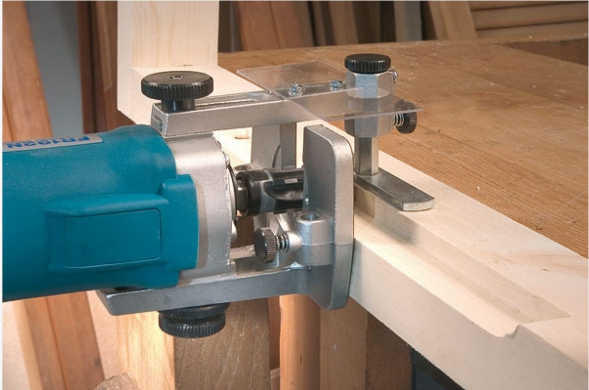
Réalisation de feuillures avec la fraise réf. 1240046 et les patins réf. 1250041 ou 1850042)
